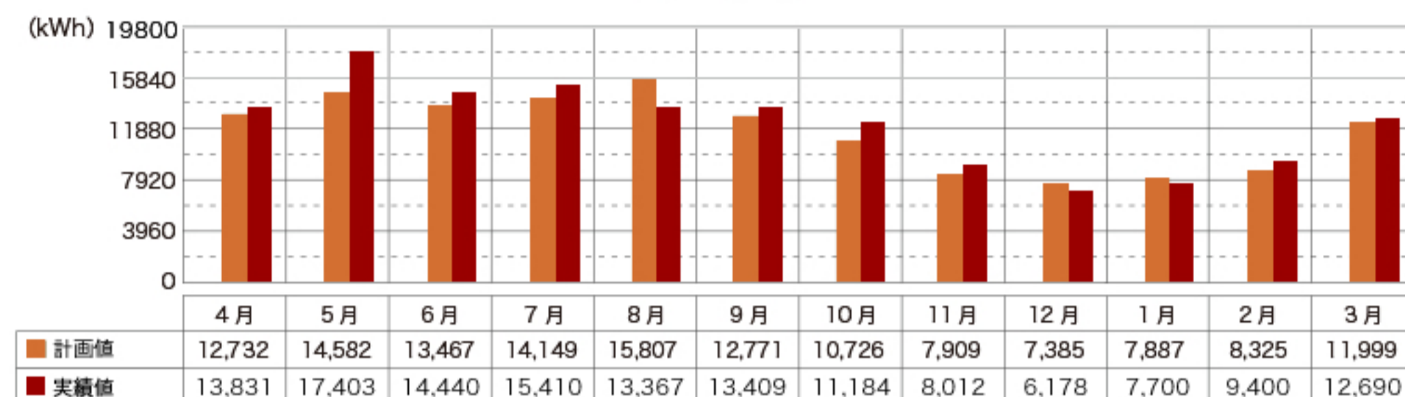
発電量 (kWh)
